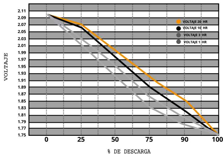
VOLTAJE VS. % DE DESCARGA
